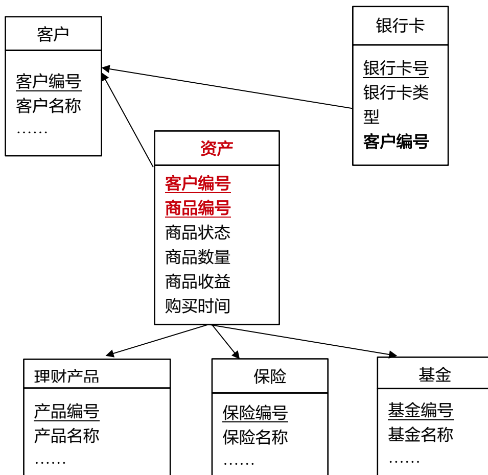
图5-2 金融数据关系模型设计图
