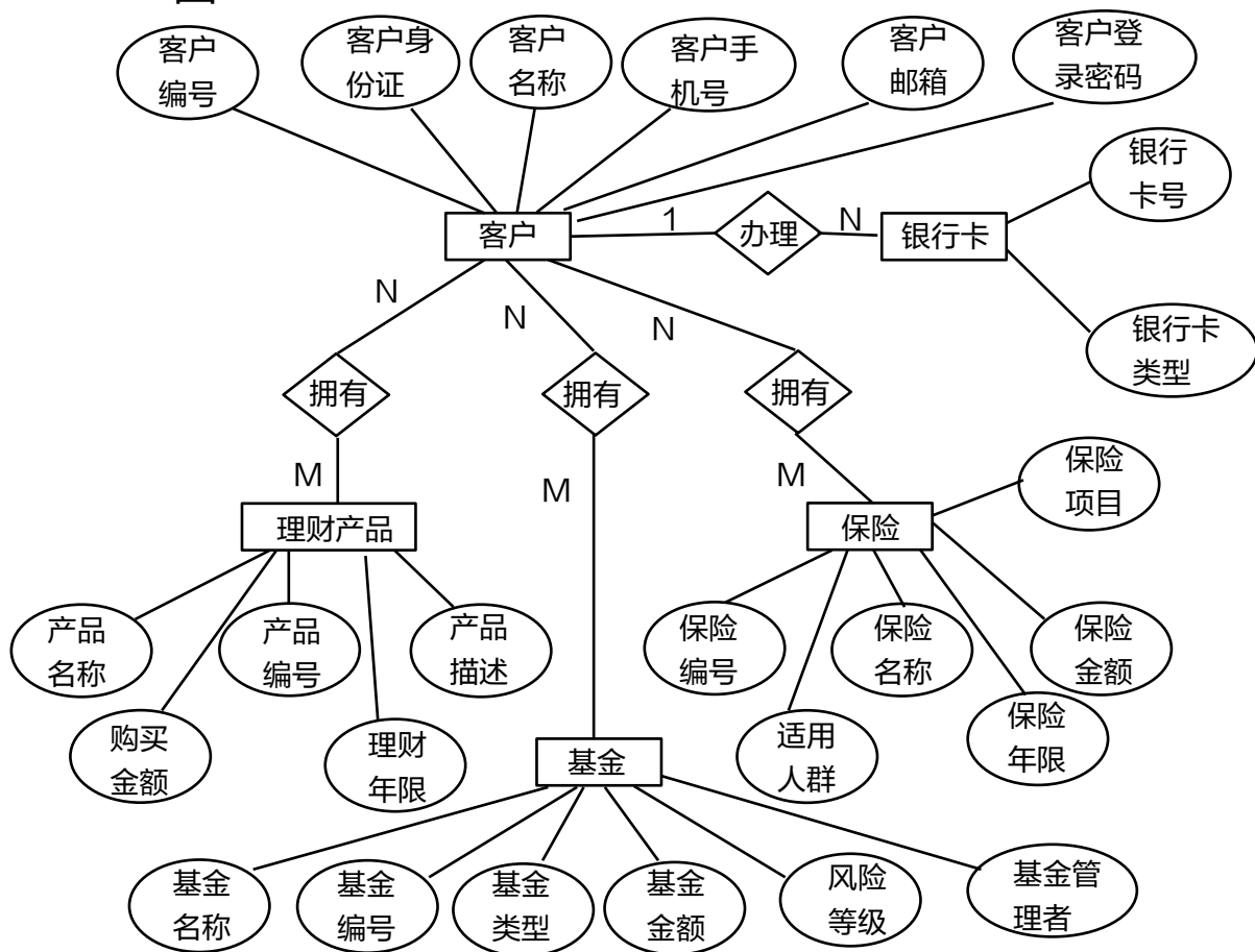
图5-1 E-R 图
